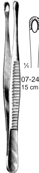
Russ. Modell 07-248-15 - 07-248-25
