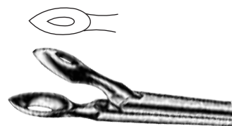
Weil 39-161-12 19 cm / 7½"
