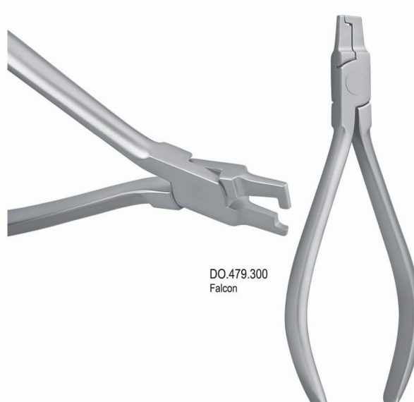
Band crimping plier Kleszcze do zaciskania pierścieni
