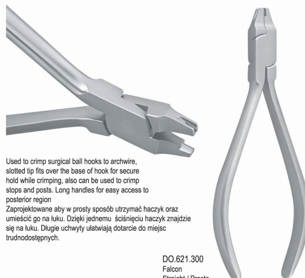
Surgical ball hook crimping pliers Kleszcze do zaciskania haczyków
